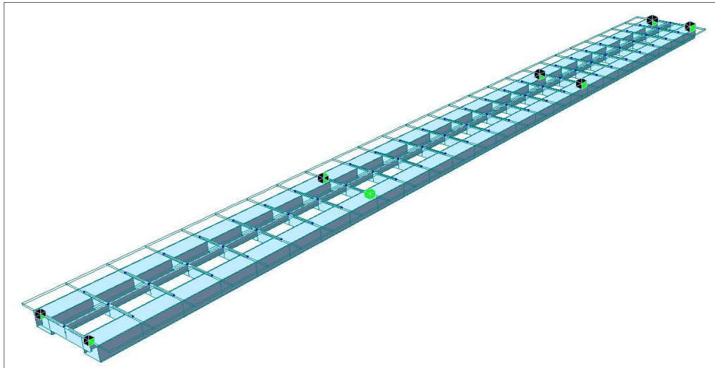
【그림 5.2】강박스 거더 구조해석 모델
