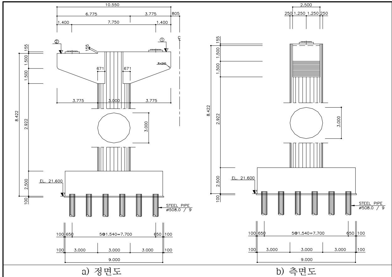
【그림 5.5】 해석단면
