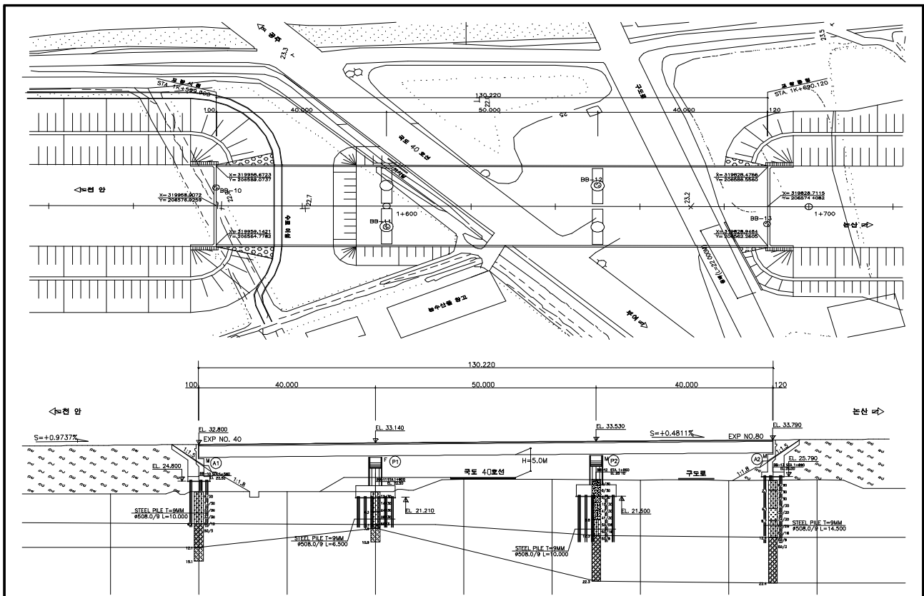
【그림 5.1】 중 · 평면도
